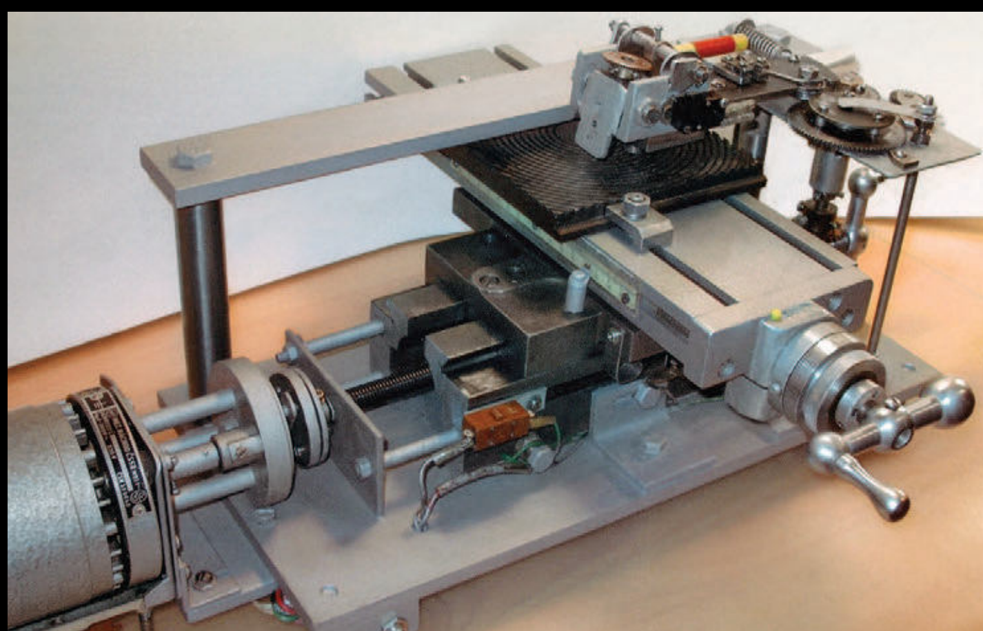
Гильошировочный станок
