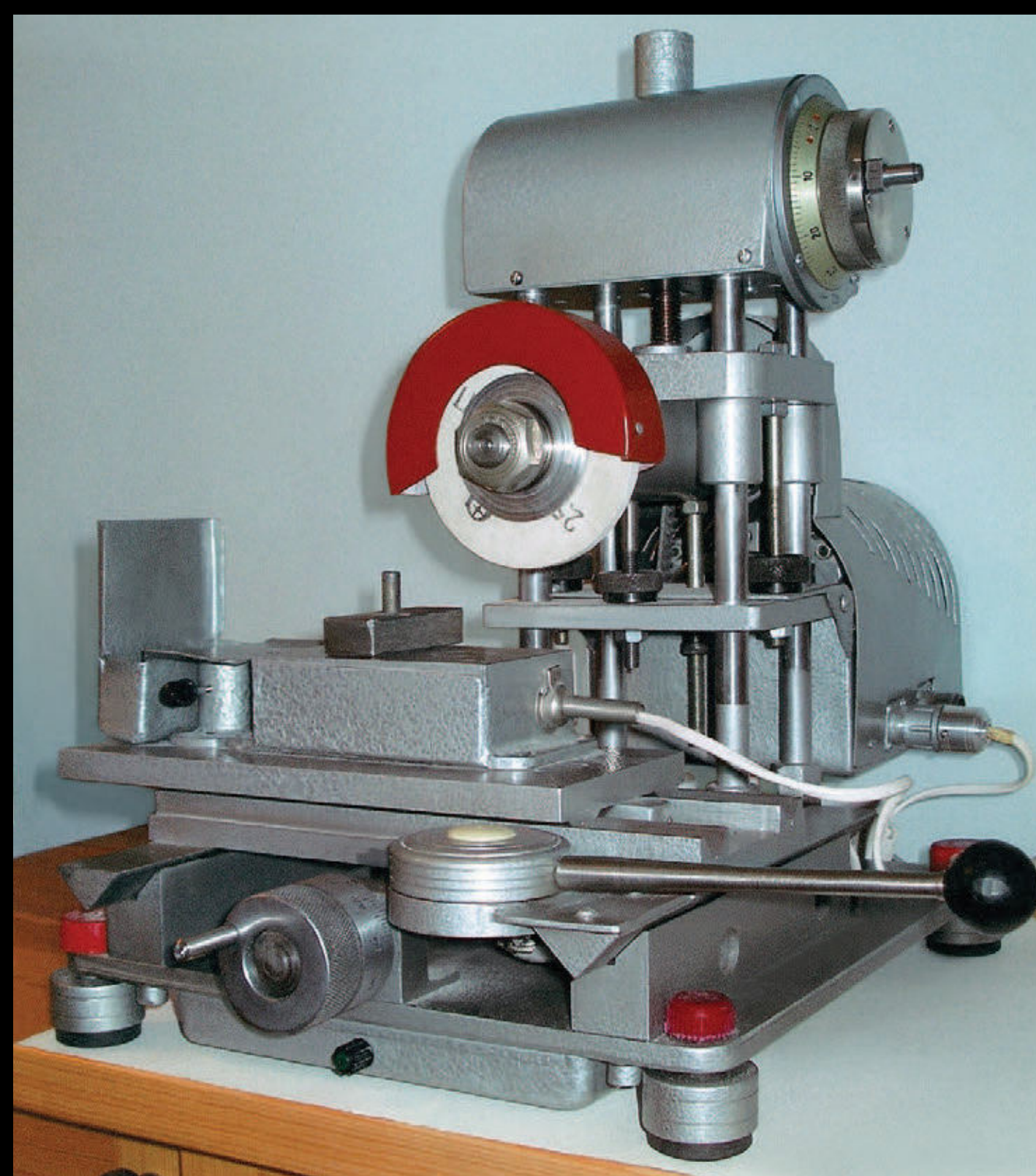
Шлифовальный станок
